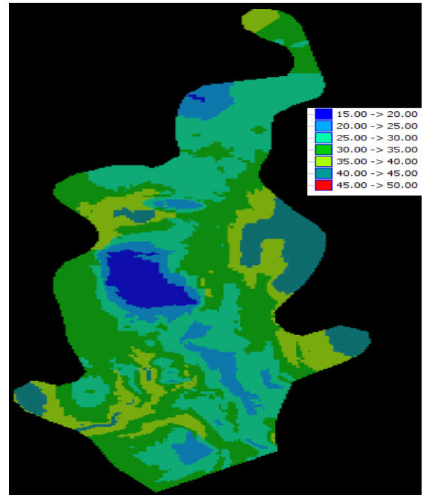
Fig. 17 % Moisture distribution.
